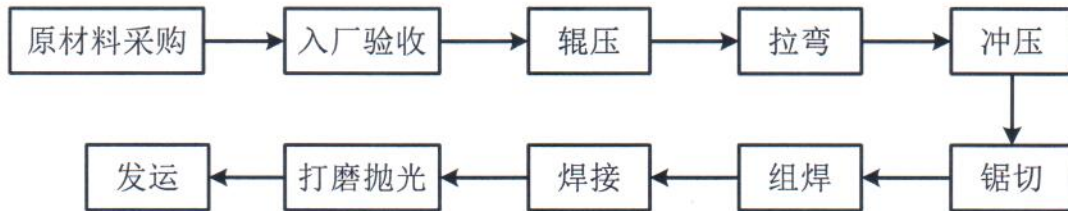
图1 车门框加工生产工艺流程图
