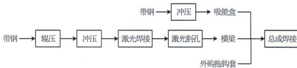
图2 保险杠生产工艺流程图
